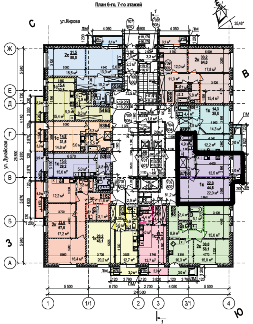
Экспликация к поэтажному плану здания (строения)
